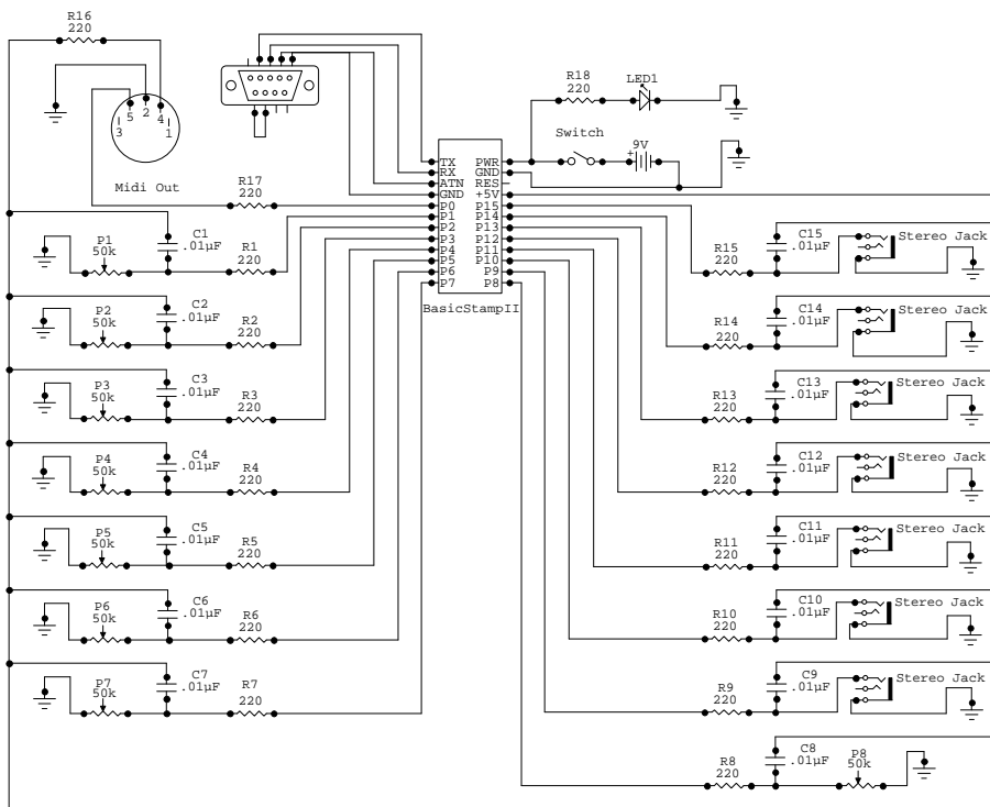
Digrama del Controlador MIDI GAB Versión: 1.0 Autor: Hugo Solís García Fecha: 25 de octubre del 2001
